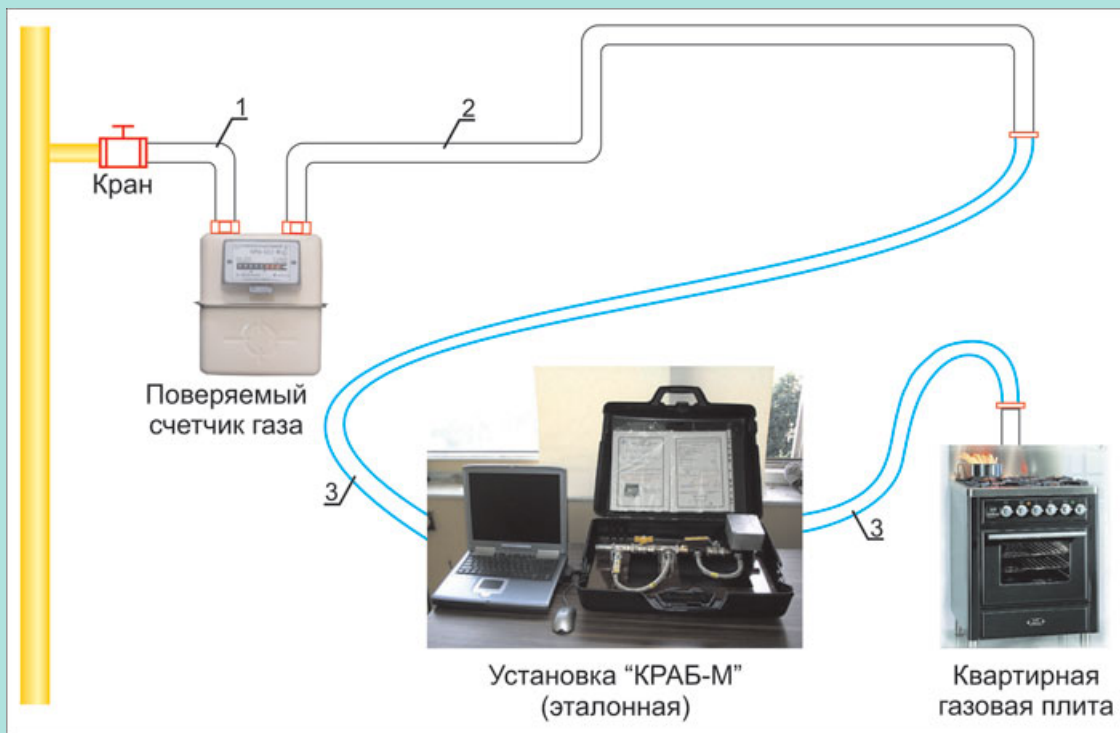
Схема подключения эталонной установки «КРАБ-М» для поверки счетчиков на месте эксплуатации
